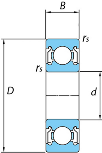
Shielded type (ZZ)
